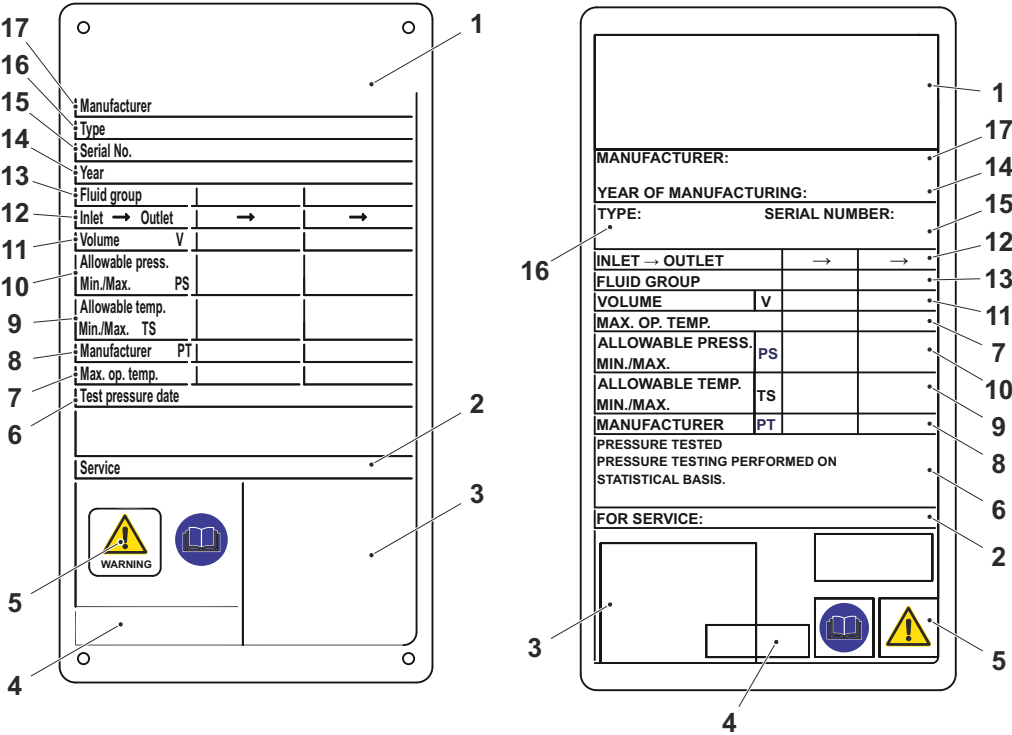
Beispiele für Typenschilder.
