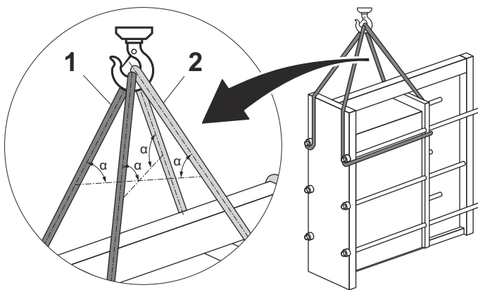
Abbildung 2: Die Abbildung zeigt die Einfädelung der Hebegurte an einem Ausrüstungsbeispiel.
