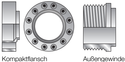
Kompaktflansch
