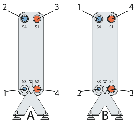
Abbildung 5: Einkreiser: A Verdampfer, B Kondensator 1.Kältemittelleintritt 2.Kältemittelaustritt 3.Wasser-/Soleeintritt 4.Wasser-/Soleeaustritt
