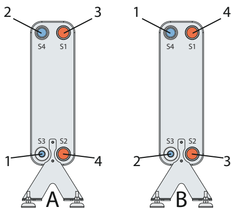
Abbildung 5: Einkreiser: A Verdampfer, B Kondensator 1.Kältemittelintritt 2.Kältemittelaustritt 3.Wasser-/Soleeintritt 4.Wasser-/Soleaustritt
